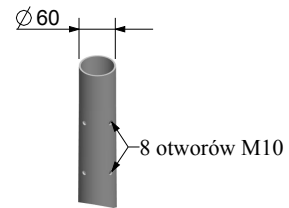
KOŃCÓWKA SŁUPA 3
