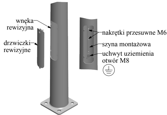
WNĘKA REWIZYJNA 2
