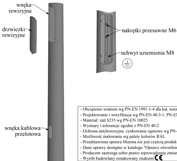
WNĘKA REWIZYJNA
