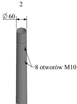
KOŃCÓWKA SŁUPA
