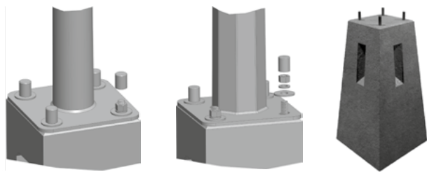
Montaż stupa do fundamentu / Pole mounting on the foundation
