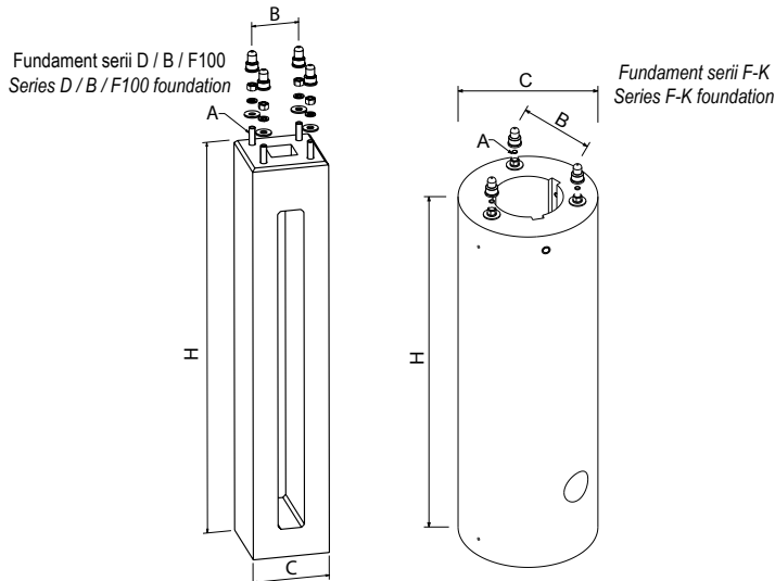
Montaż stupa do fundamentu / Pole mounting on the foundation
